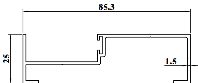
SSD749K WEIGHT : 0.666 KG/M AP : 334.35mm
