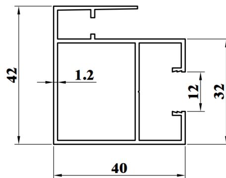
SSD752G WEIGHT : 0.636 KG/M AP : 296.19mm
