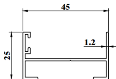
SSD750G WEIGHT : 0.374 KG/M AP : 231.23mm
