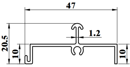
SSD915G WEIGHT : 0.308 KG/M AP : 180.89mm
