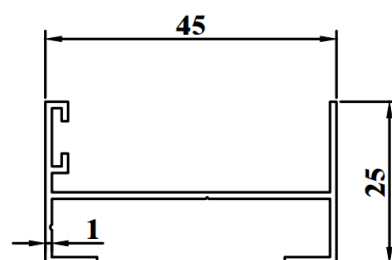
SSD750C WEIGHT : 0.314 KG/M AP : 234.21mm
