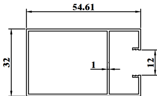
SSD754C WEIGHT : 0.520 KG/M AP : 252.85mm
