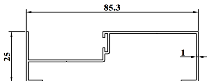
SSD749C WEIGHT : 0.454 KG/M AP : 337.96mm
