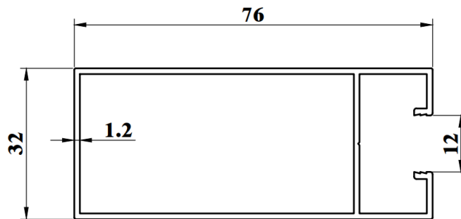
SSD797G WEIGHT : 0.763 KG/M AP : 293.21mm
