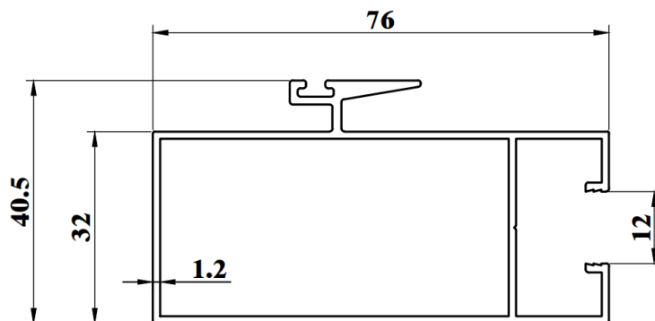
SSD798G WEIGHT : 0.915 KG/M AP : 356.50mm
