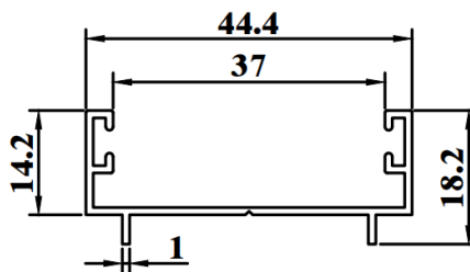
SSD755CB WEIGHT : 0.260 KG/M AP : 192.31mm
