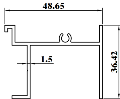
SSD746K WEIGHT : 0.548 KG/M AP : 274.43mm
