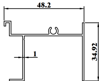
SSD746C WEIGHT : 0.370 KG/M AP : 271.49mm
