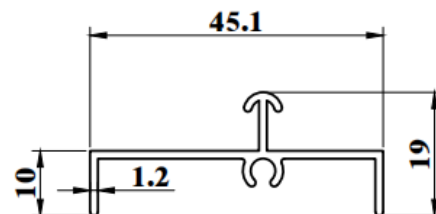
SSD748G WEIGHT : 0.283 KG/M AP : 171.77mm
